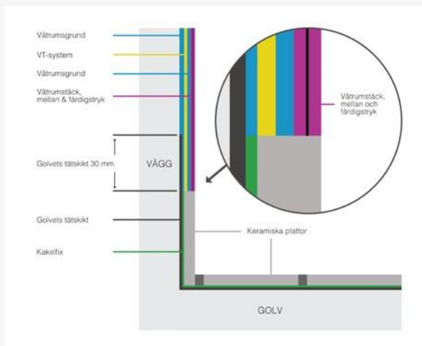
Figur 9 Figur 9 Instruktion för anslutning till keramiska plattor. Med VT-system menas i detta fall armerande material t.ex vårumsväv. Observera att i verkligheten så blir det målade våtrumssystemet inte så tjockt som det ser ut att vara i denna figur.
