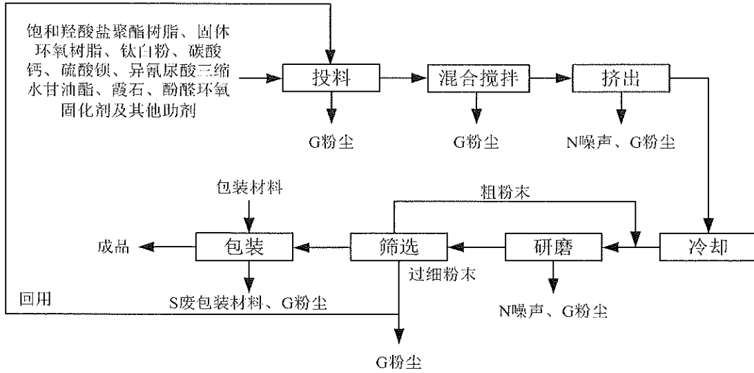
粉末涂料生产工艺流程图
